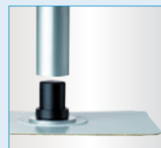
Adaption am Fahrzeugboden über selbstklebenden Flausch, Klettmatte mit Zapfen, Bodensteckteil und Distanzrohr
